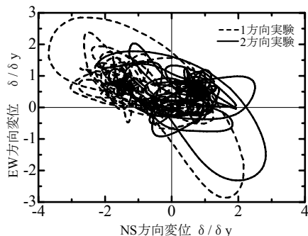
図-3 水平変位軌跡
