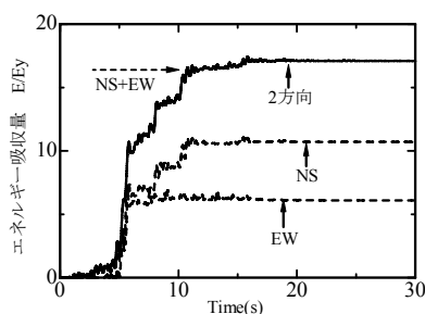
図-4 累積エネルギー吸収時刻歴曲線
