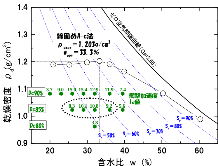
図-4 インパクト値 ( I_a ) の測定値
