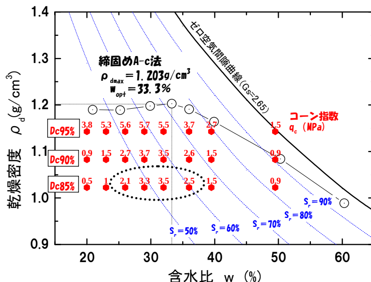
図-3 コーン指数の測定値
