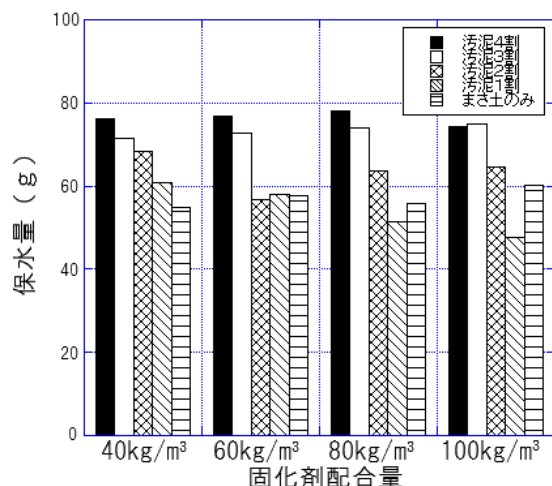
図 - 4 汚泥の有無による固化剤と保水量の関係
