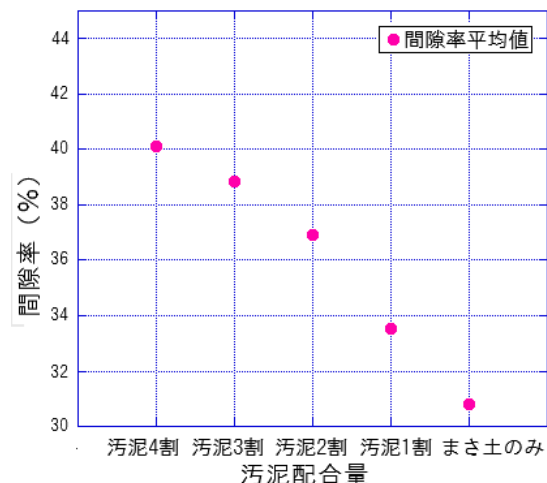
図 - 5 汚泥の配合量と間隙率の関係
