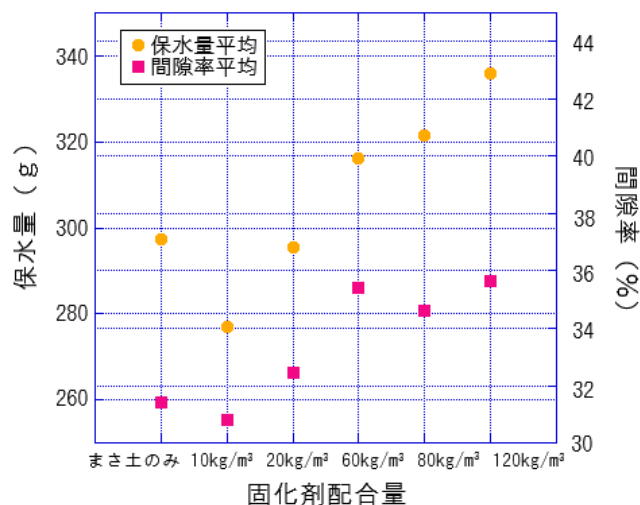
図 - 3 1 日水に浸けた場合の固化剤と保水量・間隙率の関係
