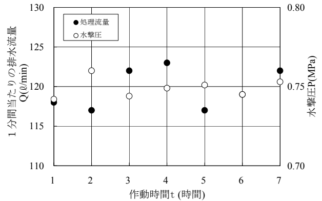
図-3 連続作動時の安定性
