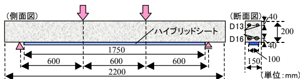
図-6 RC 梁試験体の詳細寸法
