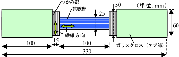
図-2 引張試験片の詳細寸法
