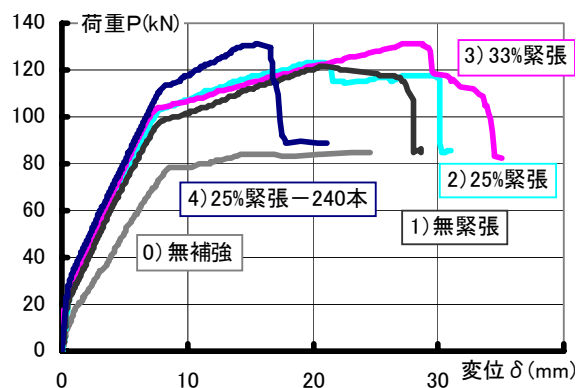
図-7 荷重-変位の関係（4点曲げ試験）
