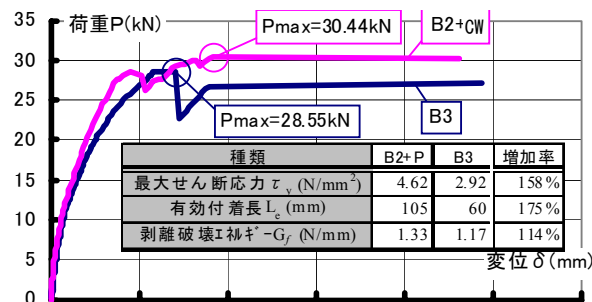
図-5 荷重-変位の関係（両引きせん断試験）
