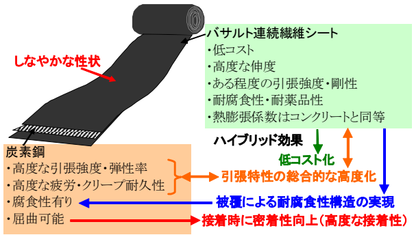
図-1 FRP-鋼線ハイブリッド構造形式の概念図
