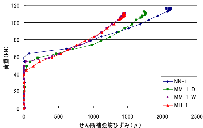
図-3 荷重－せん断補強筋ひずみ関係
