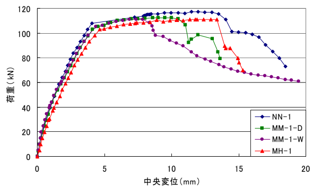
(b) せん断補強筋を有する供試体
