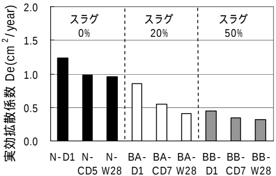
図-1 実効拡散係数 (電気泳動試験)
