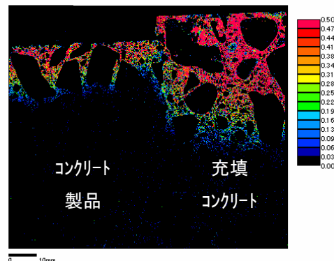
図-4 EPMA による塩素の面分析結果
