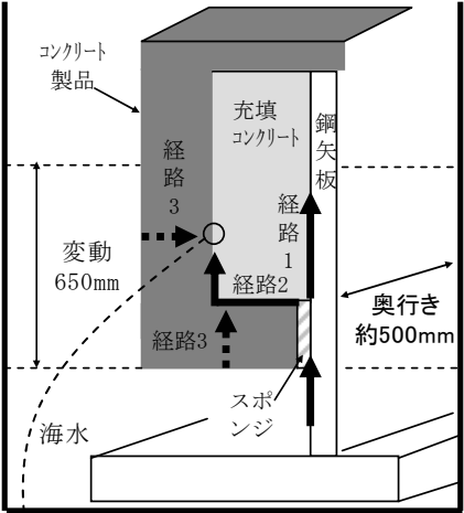
図-1 暴露供試体
