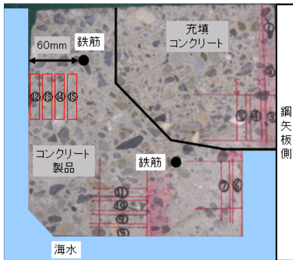
図-3 塩化物イオン濃度分析箇所
