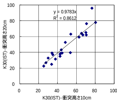
図-2 衝突高さと測定値
