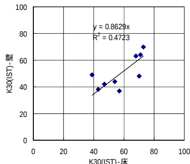
図-4 壁-床近接位置での測定値
