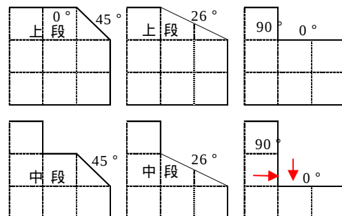
図-1 模型地盤概略(断面図:1マス=1m)
