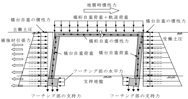
図3 作用のイメージ図 (L2地震時)
