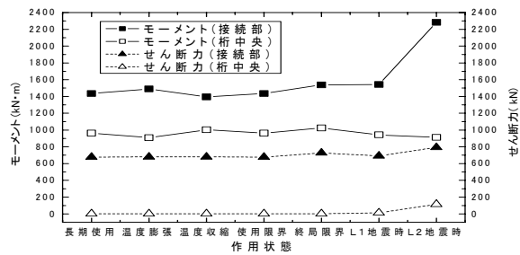
図4 作用状態と断面力の関係図
