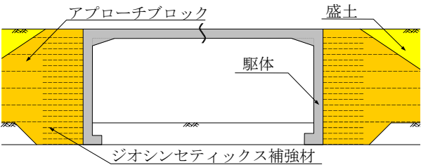
図 1 GRS 一体橋梁概要図
