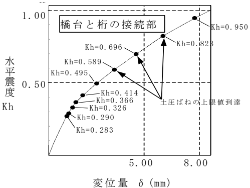
図6 水平震度～変位図
