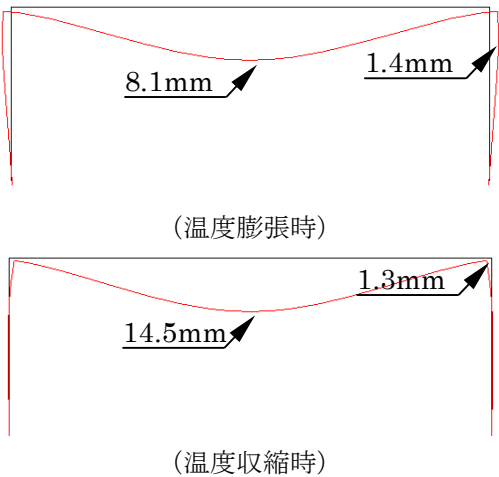
図5 温度変化考慮時の変位図
