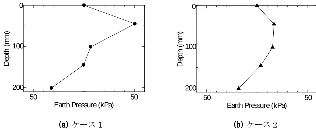
図-6 土圧分布図
