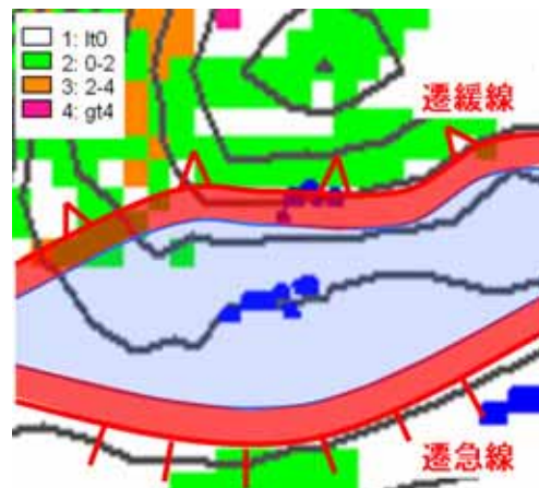
図-4 抽出箇所の崩壊危険度評価図
