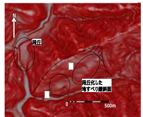
図-2 抽出する安定地形
