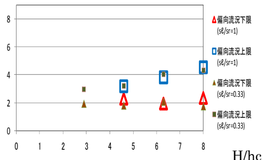
図2 c) b/B=0.125 隔壁がない場合
