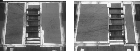
a) S_0/S_r = 1.00 の場合 b) S_0/S_r = 0.333 の場合 ( b/B=0.25 )
