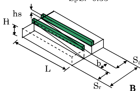
図2 d) b/B=0.125 , 隔壁がある場合 S_0/S_r=0.33
