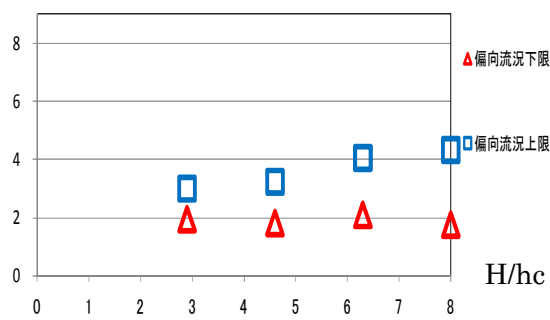
図2 d) b/B=0.125 , 隔壁がある場合 S_0/S_r=0.33
