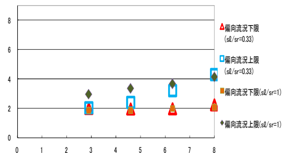
図2 b) b/B=25 , 隔壁がある場合
