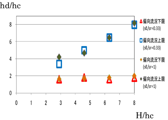
図 2 水衝部を伴う偏向流況の形成領域 a) b/B=0.25 隔壁がない場合
