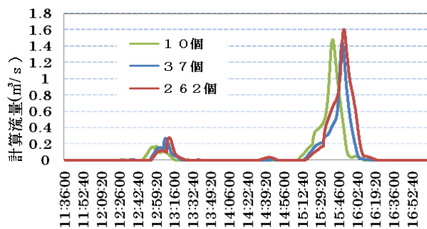
図3 支流域分割数別の流出特性比較結果
