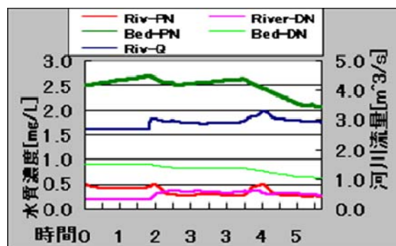
図4 河川・河床間隙水水質解析結果
