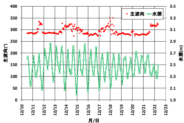
図-4 主波向と水深
