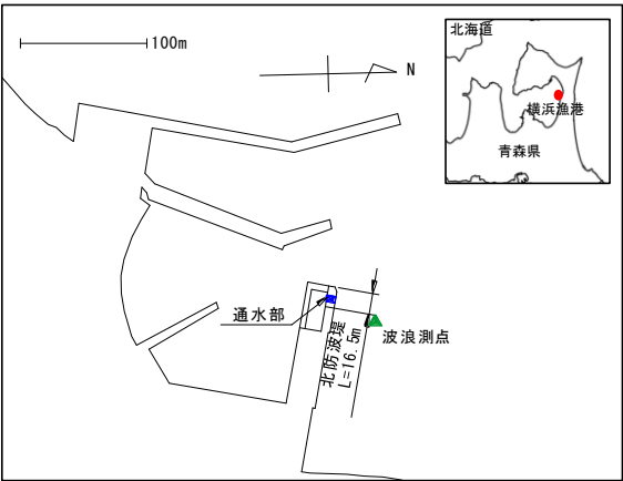
図-3 青森県横浜漁港の平面図
