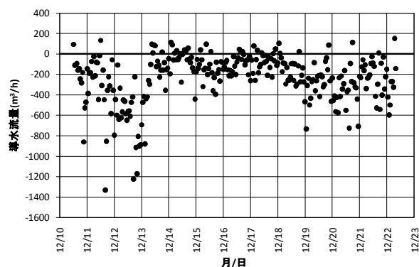
図-6 遊水室型防波堤の導水流量
