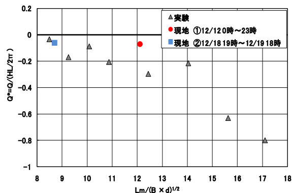
図-7 実験と現地との導水量の比較
