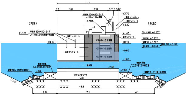
図-2 源氏ヶ浦漁港北防波堤標準断面図
