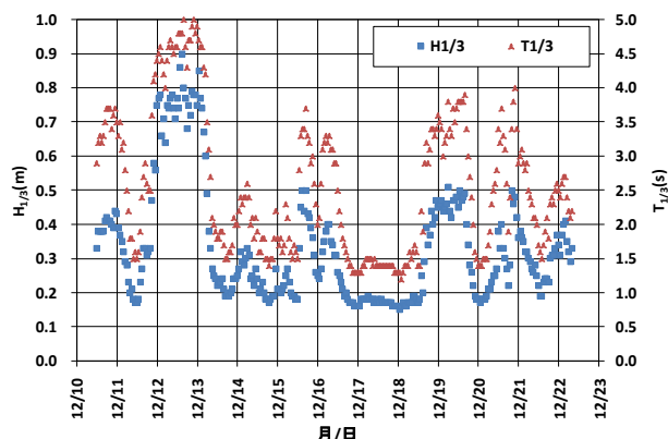
図-5 有義波高 H_{1/3} と有義波周期 T_{1/3}
