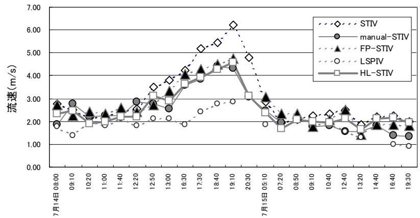
図-3 流速結果
