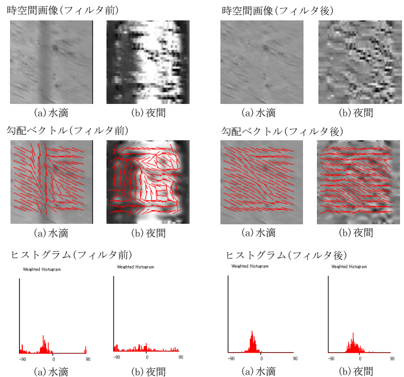
図-4 バンドパスフィルタ適用による変化
