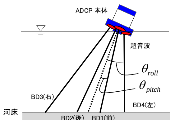
図-1 ADCP を搭載したボートの揺動が計測値に与える影響
