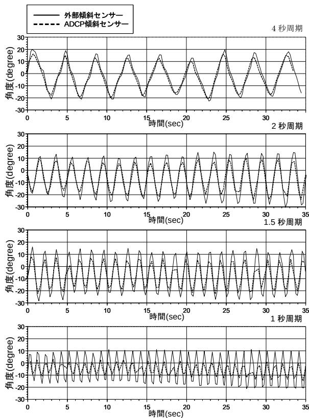
図-2 ADCP と外部傾斜センサーのピッチ角計測値の比較
