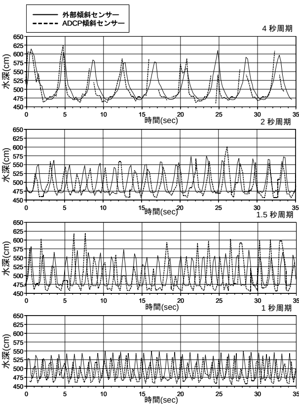
図-3 ADCP と外部傾斜センサーの水深(BD3)の比較
