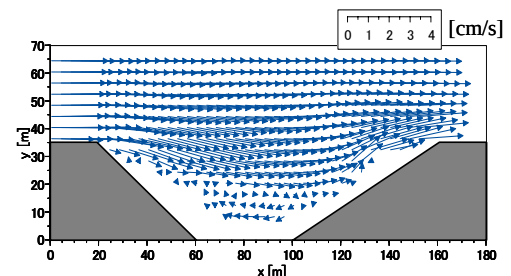
図-5 流速ベクトル(数値計算)
