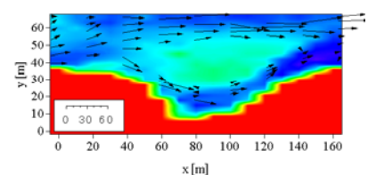
図-2 流速ベクトル(実測)
