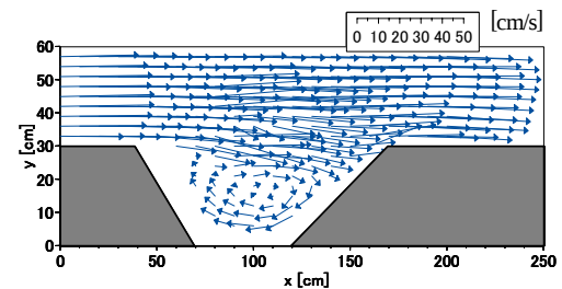
図-3 流速ベクトル(実験)
