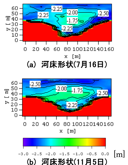
図-1 河床変動コンター
