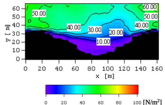
図-6 底面せん断応力分布(数値計算)
