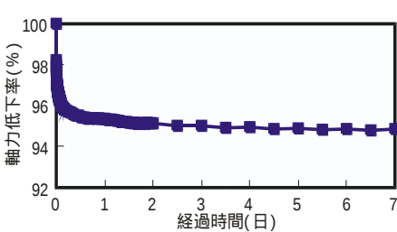
図 - 1 リラクゼーション試験
