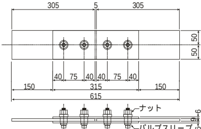
図 - 2 試験体形状
