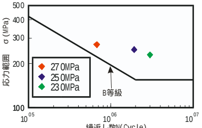
図 - 4 疲労試験結果
