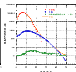
図8 対象海域における風速の出現頻度分布
