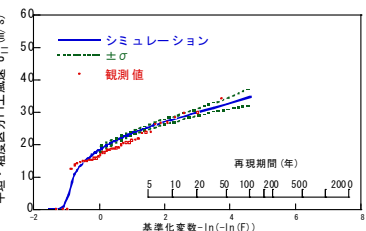
図6 台風による風速の際威厳期間別期待値
