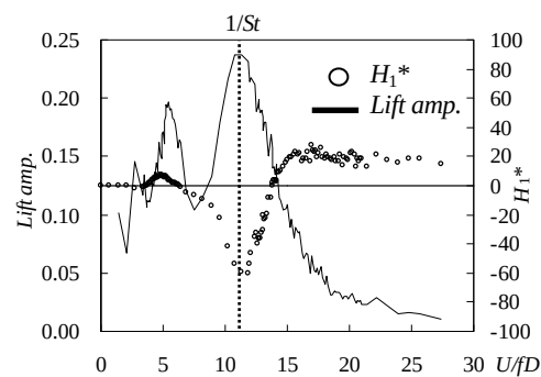
Fig.3 B/D=2 における揚力の振幅 (スプリッタープレート無、 2\eta/D=0.025 、一樣流)
