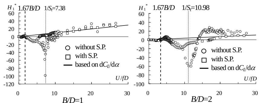
Fig.1 B/D=1, 2 における非定常空気力係数 H_1^* ( 2\eta/D=0.025 , 一様流)
