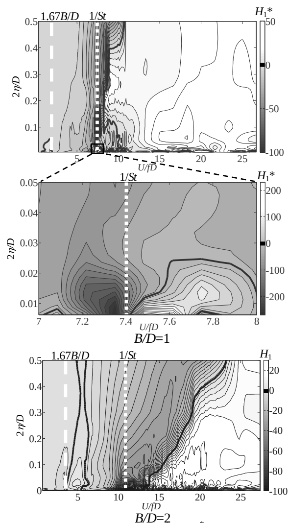
Fig.2 風速-振幅- H_1^* 図 (スプリッタープレート無、一樣流)
