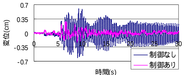
Fig.5 制御の有無による観測点3の応答変位比較図
