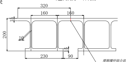
図-2 アルミニウム床版の断面
