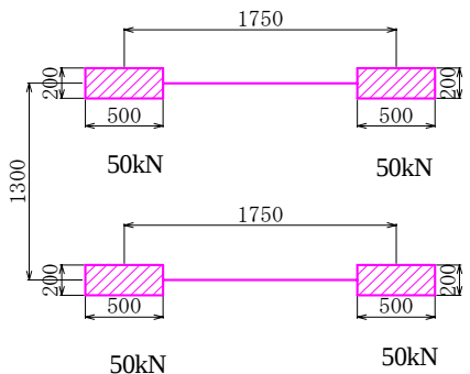
図-7 たわみ荷重
