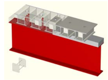
図-5 床版と鋼桁の連結構造
