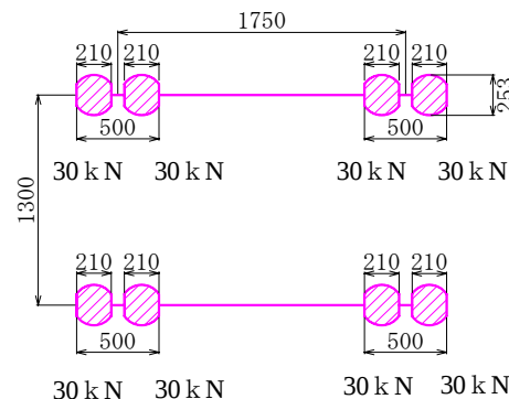
図-4 疲労荷重
