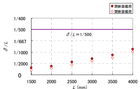
図-9 たわみと支間長の関係
