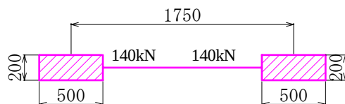
図-3 活荷重
