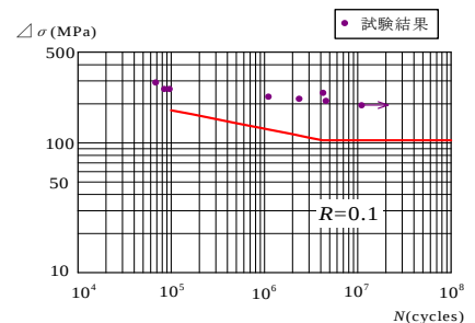
図-6 試験結果と S-N 曲線
