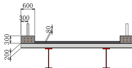
図-1 アルミニウム床版を有する道路橋の断面
