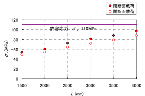
図-8 床版の上板上面の 応力と支間長の関係
