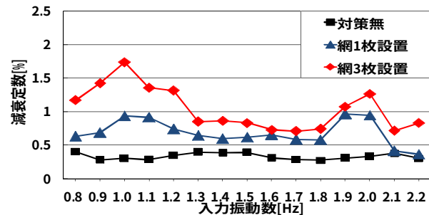
図 4 減衰定数の比較
