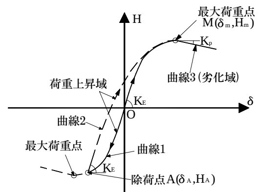
図-1 鋼製橋脚復元力履歴曲線
