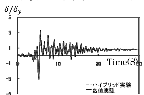
(d) 応答変位履歴(JMA-EW)
