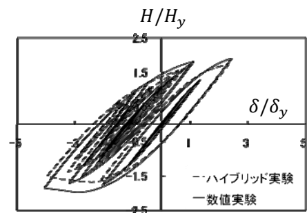
(a) 復元力-変位履歴(JMA-NS)
