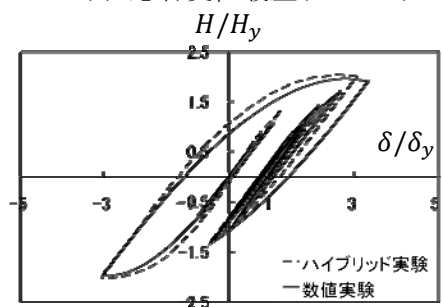
(c) 復元力-変位履歴(JMA-EW)
