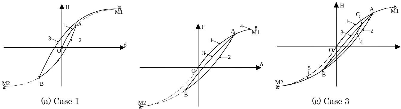
図-2 除荷一再加荷時の履歴
