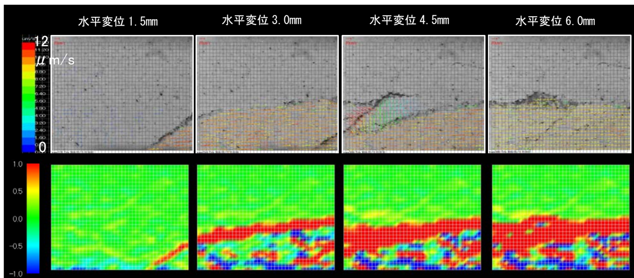
図3 正規圧密供試体のせん断過程におけるせん断帯の観察： (a)速度ベクトル(上図)，(b)せん断ひずみ(下図)
