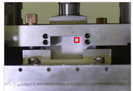
図1 せん断帯観察用せん断箱 (赤枠部分はマイクロスコープ で観察する領域)
