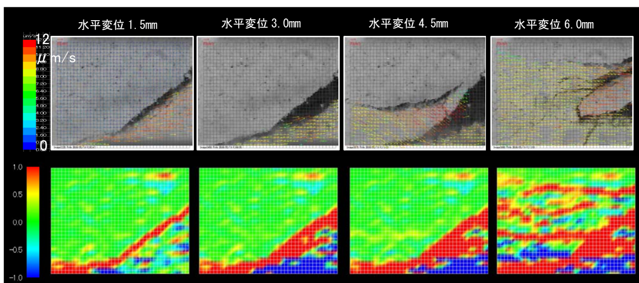
図4 過圧密供試体のせん断過程におけるせん断帯の観察： (a)速度ベクトル(上図)，(b)せん断ひずみ(下図)
