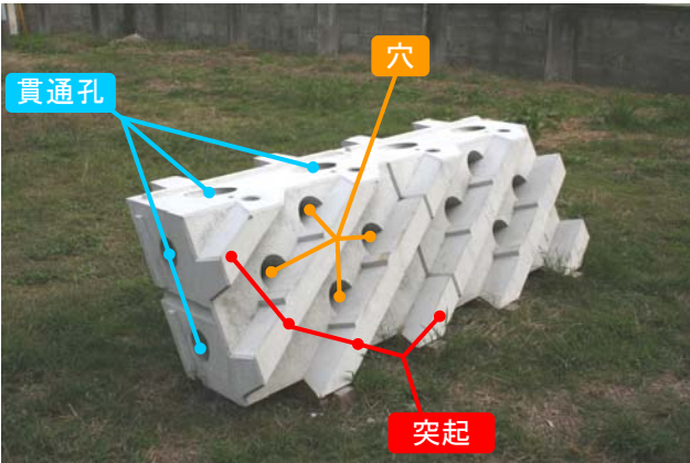
写真1 1 m 5 分勾配型ブロック構造体 (2 個のブロック構造体を並べた状態)
