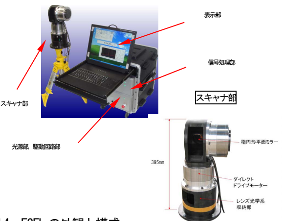
図4 FSFLの外観と構成
