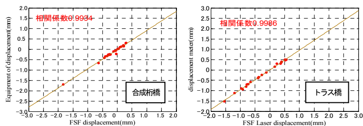
図9 たわみのピーク値の相関図
