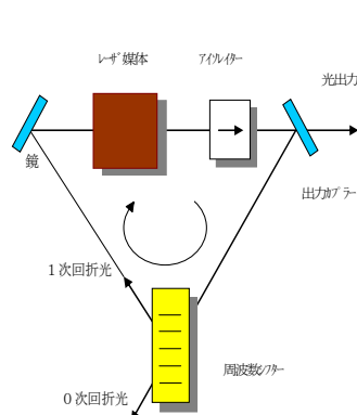
図2 FSF レーザの基本構成
