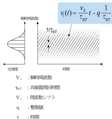
図3 チャープ周波数出力
