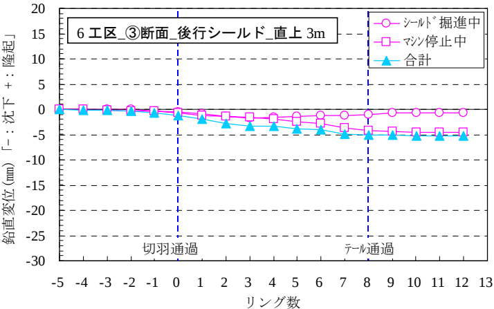
図-4 各施工段階における鉛直変位量の関係
