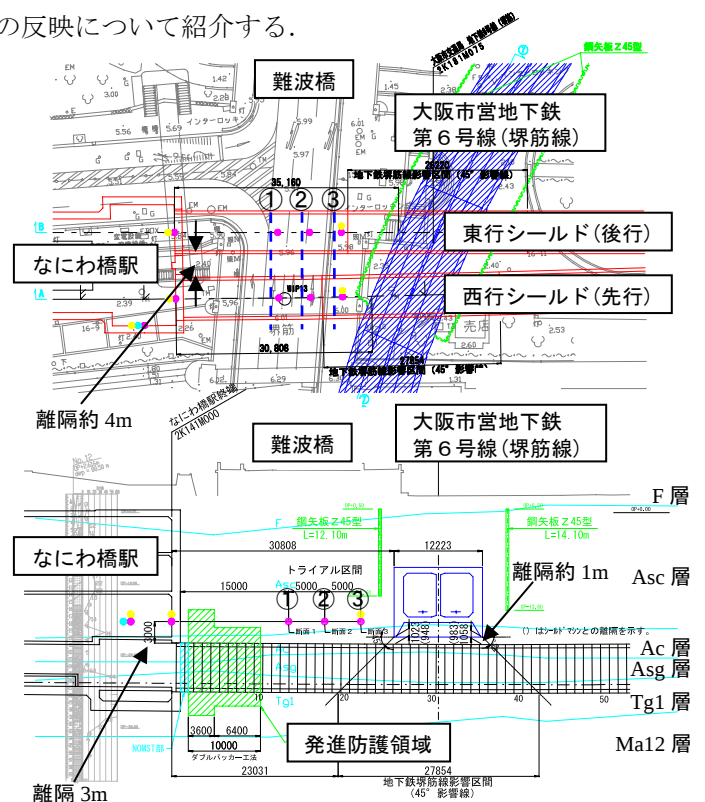
図-1 計測断面平面図および縦断面図
