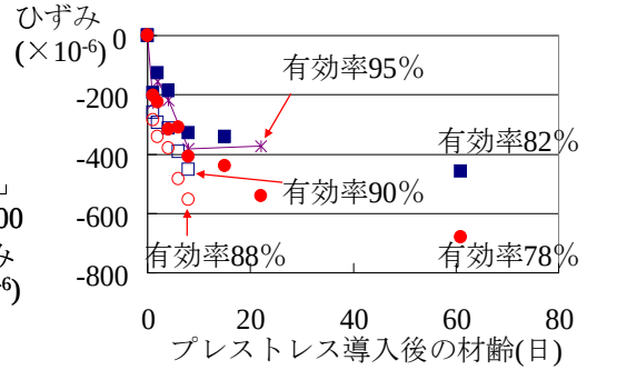
図-4 スパン中央下縁コンクリートのひずみ変化
