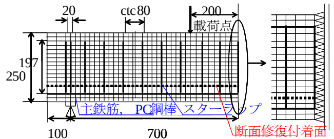
図-2 断面修復 PC 供試体解析モデル (単位: mm)
