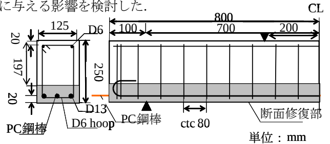
図-1 断面修復 PC 供試体の形状・寸法
