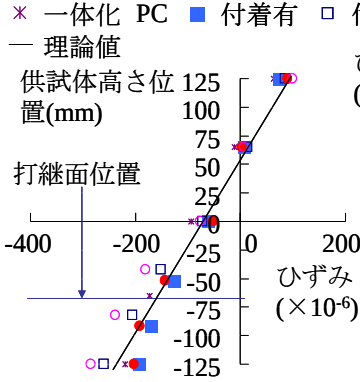
図-3 プレストレス導入時の供試体高さ方向ひずみ分布
