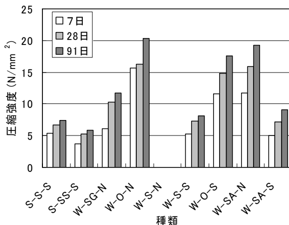
図-5 ポーラスコンクリートの圧縮強度
