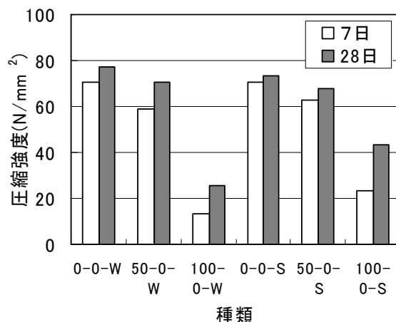
図-3 圧縮強度 (固形分無し)
