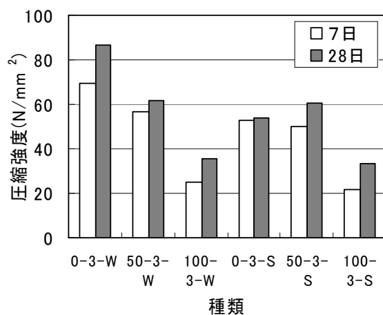
図-4 圧縮強度 (固形分有り)
