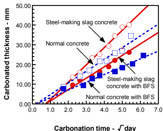
図4 骨材の種類が中性化に及ぼす影響
