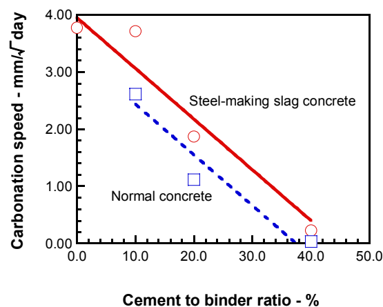
図2 セメント結合材比と中性化速度の関係
