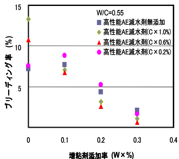
図-1 増粘剤添加率がモルタルのブリーディング率に及ぼす影響
