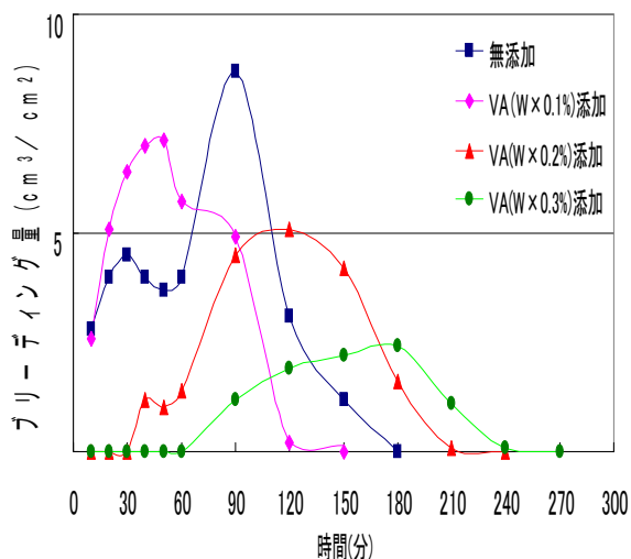
図-2 VA 添加がブリーディング発生 時間と量に及ぼす影響
