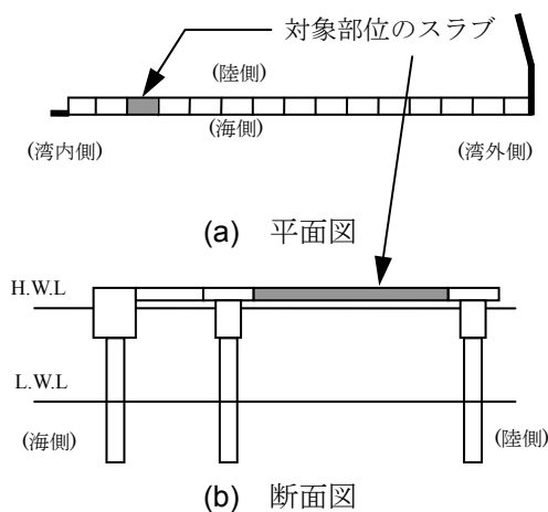
図 1 対象構造物
