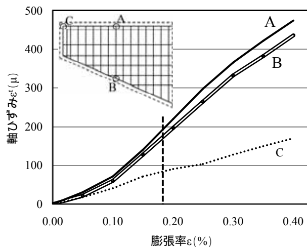
図9 鉄筋の軸応力
