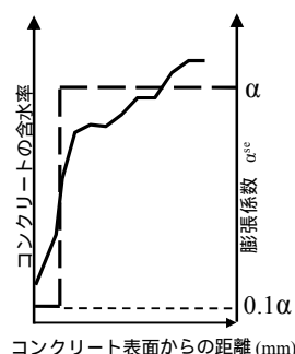
図2 コンクリートの含水率と膨張係数
