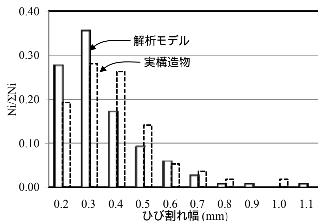
図8 ひび割れ幅分布
