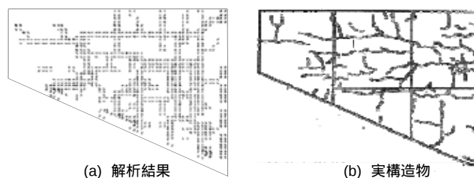
図7 ひび割れ性状比較
