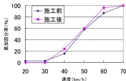
図5 車両速度の累加百分率
