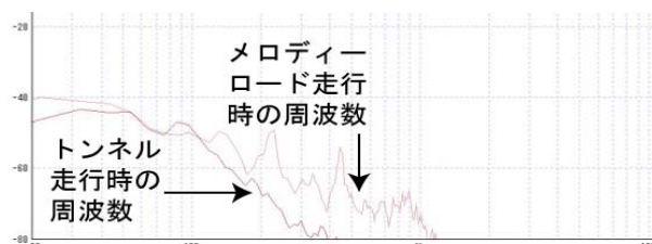
図2 周波数特性
