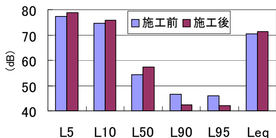
図3 トンネル脇の騒音
