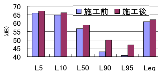
図4 車内の騒音
