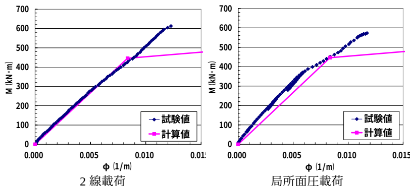
図-5 M- \phi 関係図
