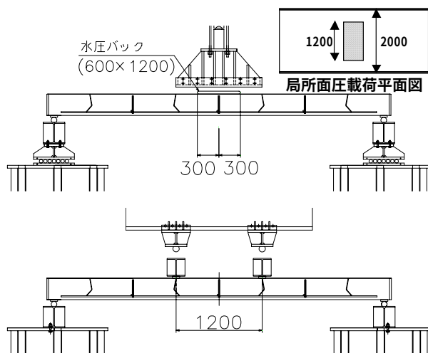
図-3 載荷概要図
