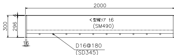
図-2 平板試験体 主断面図
