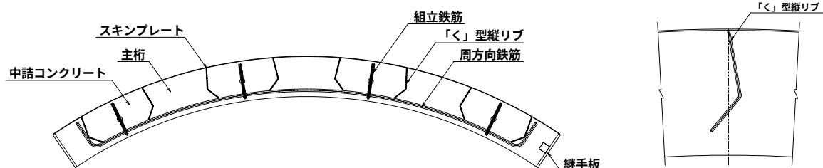
図-1 コンクリート中詰型合成セグメント構造概要図
