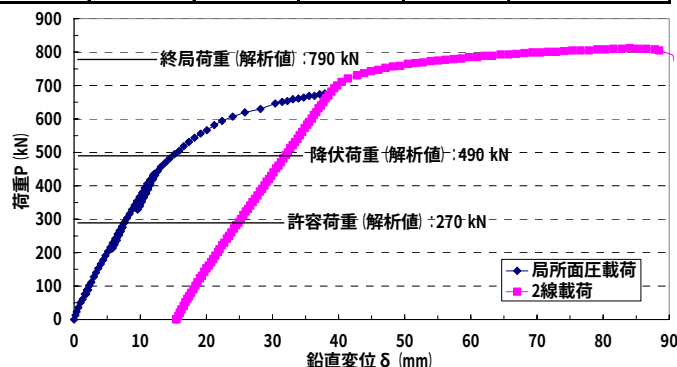
図-4 P- \delta 関係図
