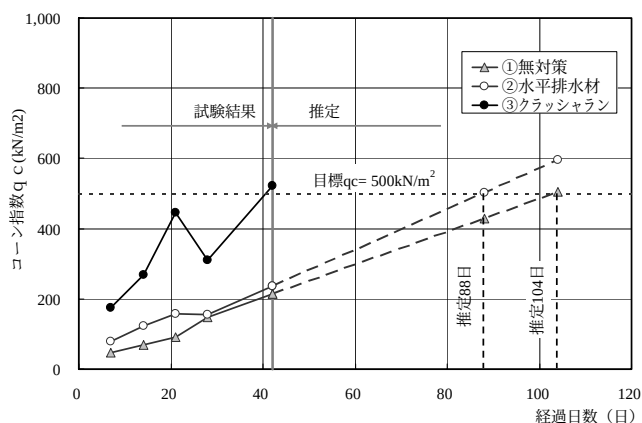
図-4 コーン指数の経時変化
