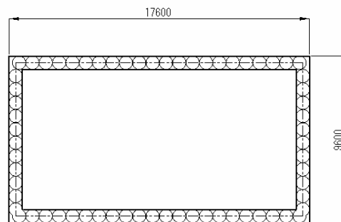
図-1 試験施工ヤード概略図
