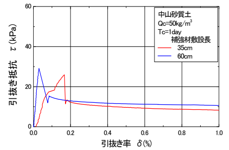
図-3 補強材の敷設長の影響
