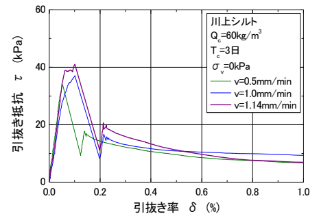
図-4 引抜き速度の影響
