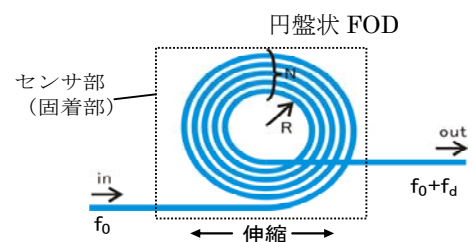
図-1 光ファイバのセンサ部模式
