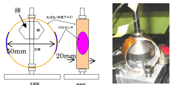
図-3 FOD 振動計の構造
