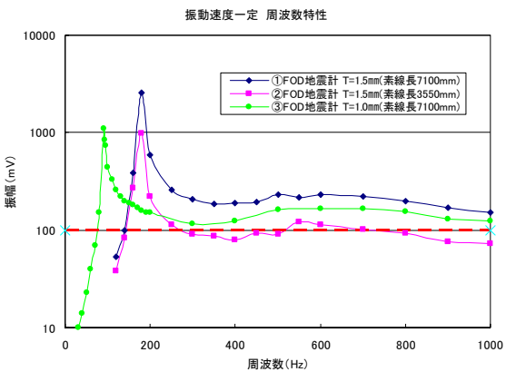
図-6 FOD センサの特性
