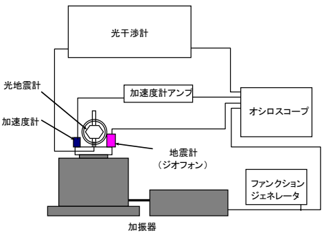
図-5 計測システム
