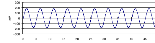
図-4 各種センサの振動波形（200Hz）
