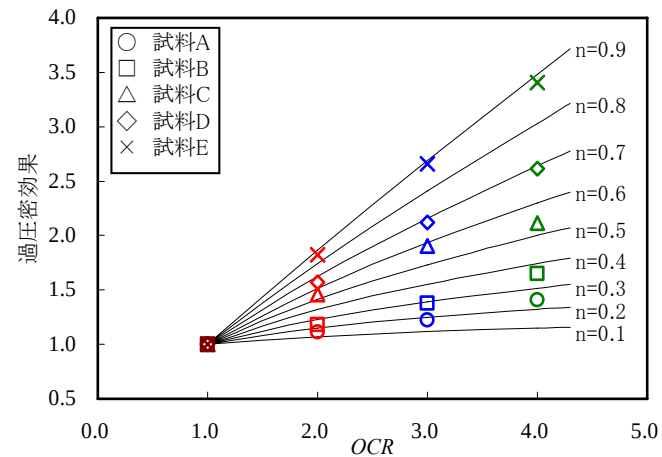
図 1 過圧密効果と過圧密比の関係
