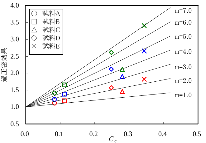
図 2 過圧密効果と圧縮指数の関係
