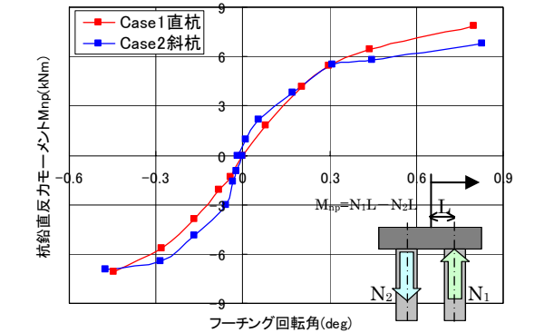
図4 杭頭鉛直反力モーメントーフーチング回転角
