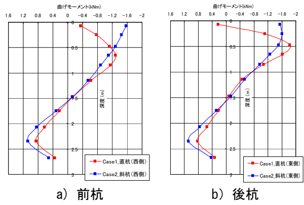
図6 地盤変位载荷_曲げモーメント分布図
