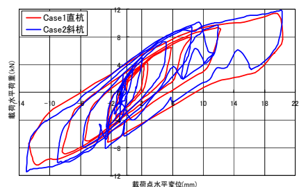
図 2 水平荷重—水平変位
