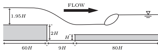
図-1 流れ概要 3)
