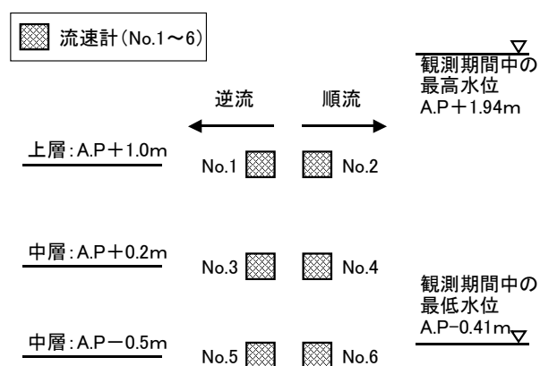
図-1 流速計の配置
