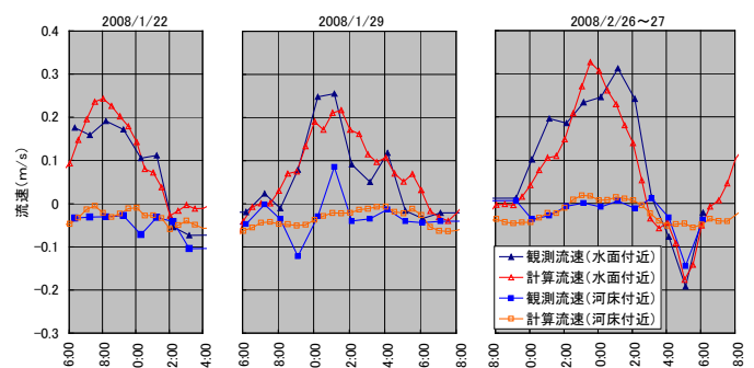
図 - 4 流速の比較
