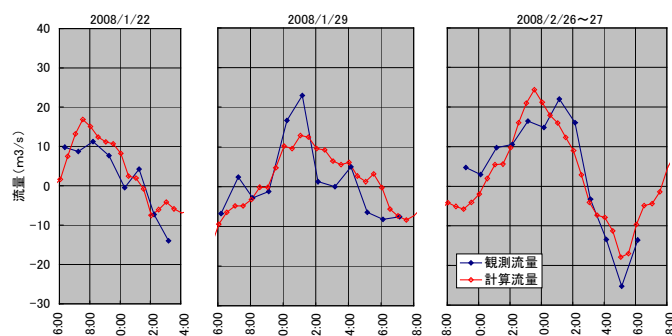
図 - 3 流量の比較
