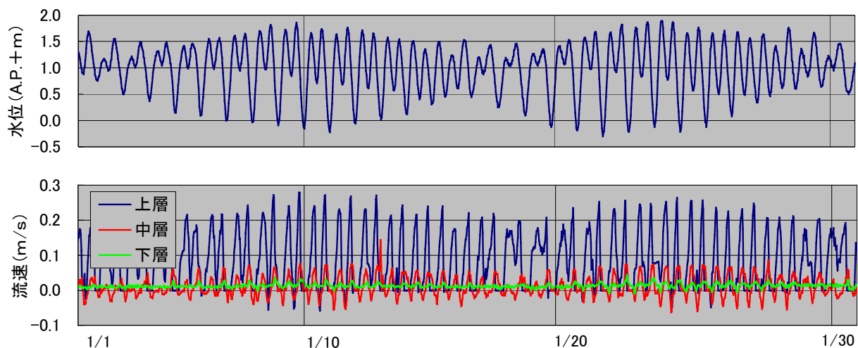
図 - 2 2008 年 1 月の水位・流速の変化
