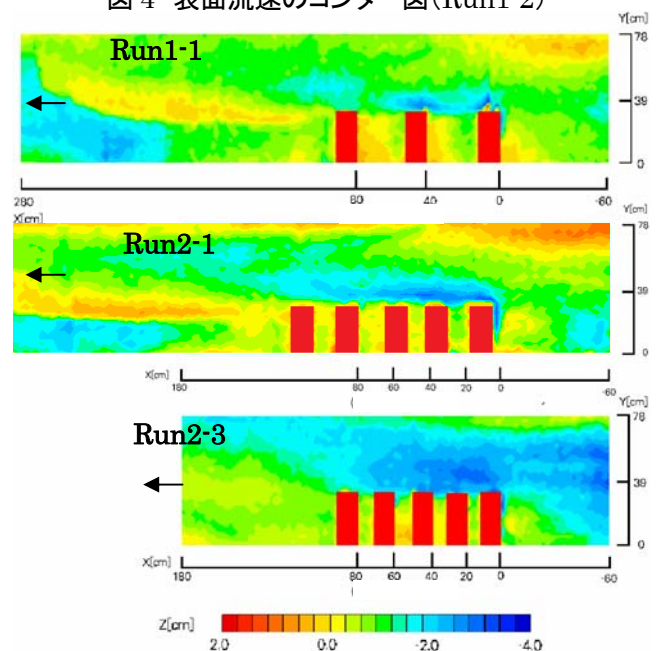
図5 河床変動量のコンター図
