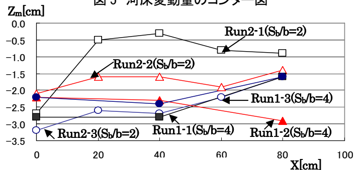
図6 置石群先端の洗掘深の流下方向分布
