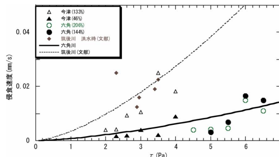
図－1 せん断応力と浸食速度の関係
