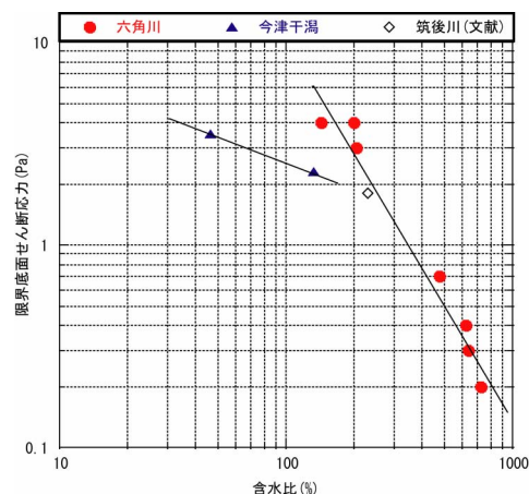
図－2 含水比と限界底面せん断応力の関係
