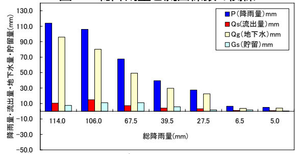
図-6 人工芝グラウンドの水収支の推定結果 地下水量は降雨強度と降雨継続時間を一致させ模型実験より算出
