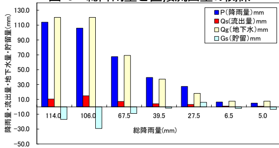
図-5 人工芝グラウンドの水収支の推定結果 地下水量は降雨強度を一致させ模型実験より算出
