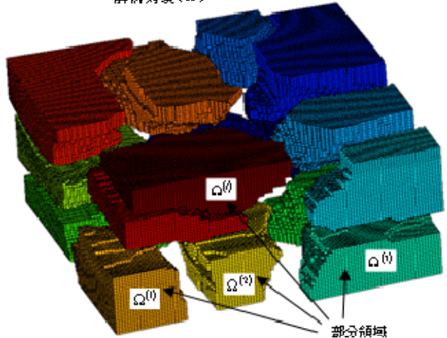
図1 並列解析のための領域分割
