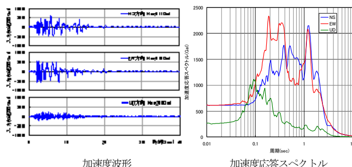
図 3 入力地震波
