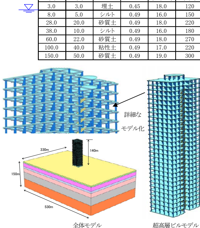
図 2 解析モデル
