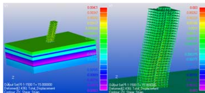
図 4 変形+せん断ひずみ分布図(15sec)
