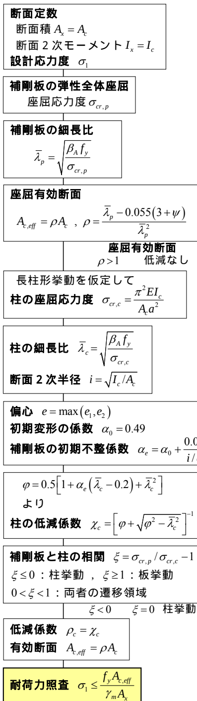
図-2 規準 A の概略フロー
