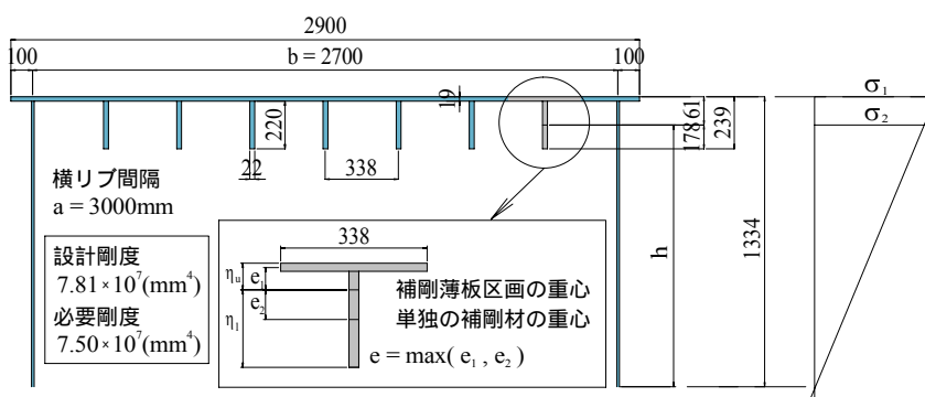
図-1 比較対象の補剛板
