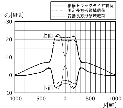
図-5 上板に生じる応力 \sigma_y の分布
